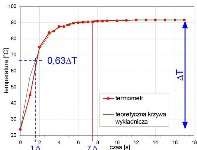
Rysunek 1. Wykres wskazań termometru w funkcji czasu podczas pomiaru temperatury wody
