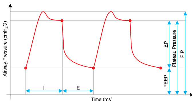
Rysunek 2. Cykl oddechowy respiratora, z zaznaczonymi kluczowymi parametrami ciśnień: dodatnie ciśnienie końcowo-wydechowe (PEEP), ciśnienie sterujące ( \Delta P ), szczytowe ciśnienie wdechowe (PIP) i ciśnienie plateau. Pokazane są również parametry czasowe wdechu (I) i wydechu (E)
